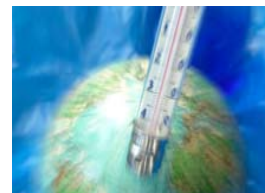
„Ozonloch und globale Erwärmung – Menschenwerk oder natürliche Fluktuation?“ Prof. Dr. Erich Übelacker
